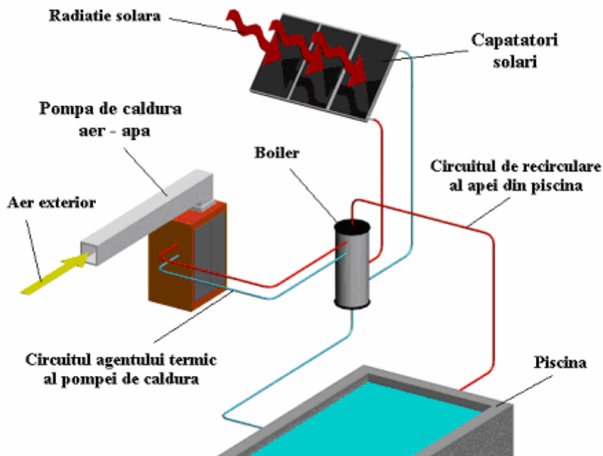
Fig. 13. Încălzirea apei din piscină cu ajutorul unei pompe de căldură aer-apă și a unor colectori solari
