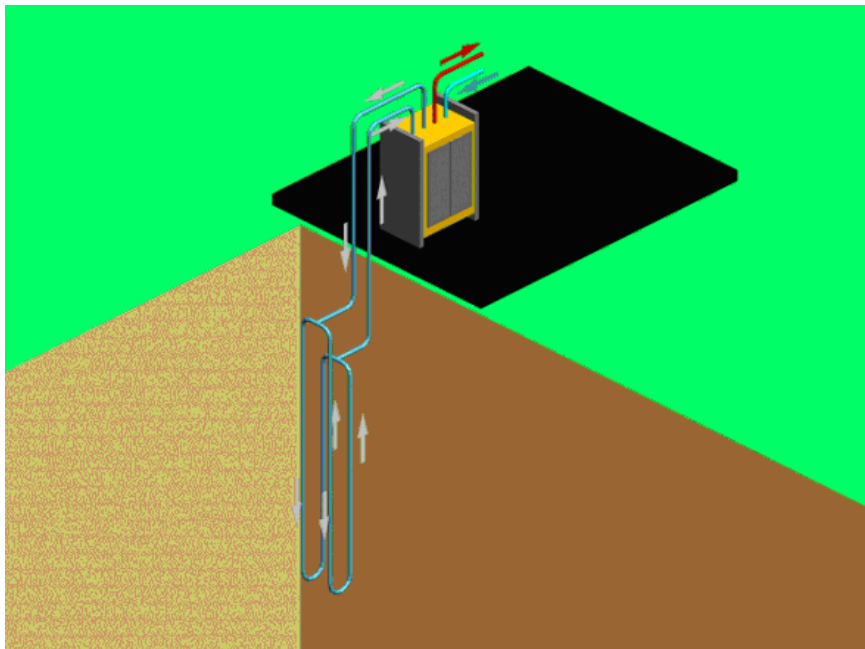
Fig. 9. Colectori verticali pentru captarea căldurii din sol
