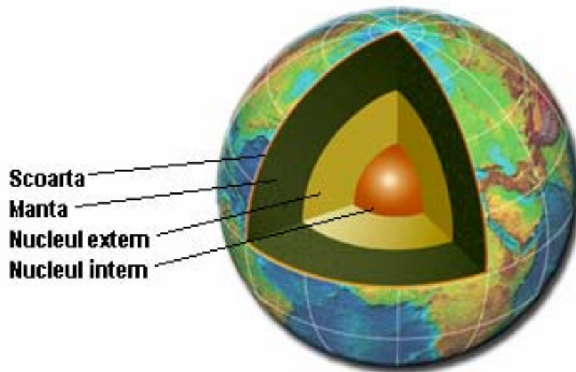
Fig. 1. Principalele zone din care este alcătuit Pământul academic.evergreen.edu
