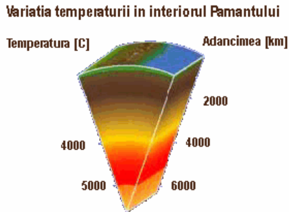
Fig. 2. Variația temperaturii dinspre scoarța spre centrul Pământului academic.evergreen.edu
