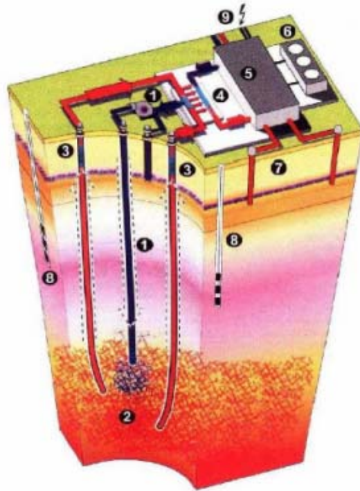
Fig. 4. Părțile componente ale unei centrale electrice geotermale
