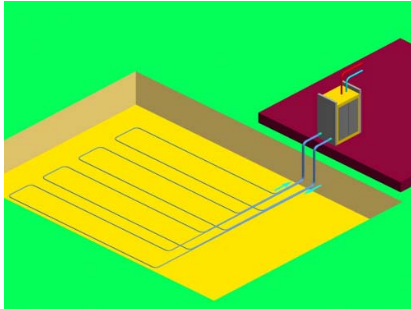
Fig. 10. Amplasarea direct în sol a vaporizatorului pompei de căldură
