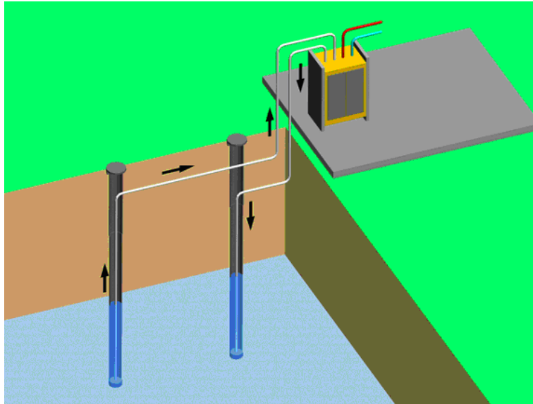
Fig. 11. Utilizarea apei freactice ca sursă de căldură
