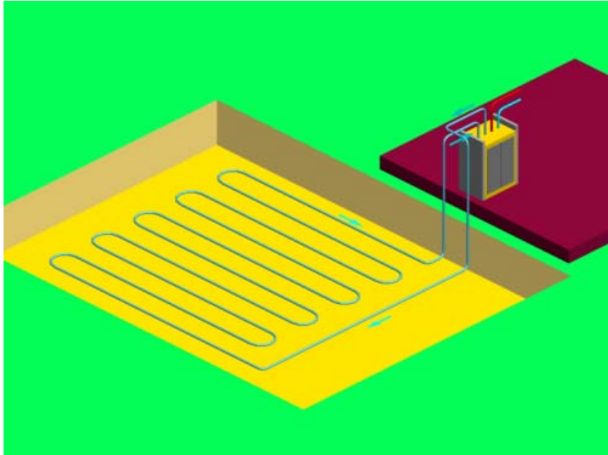
Fig. 8. Colectori orizontali pentru captarea căldurii din sol
