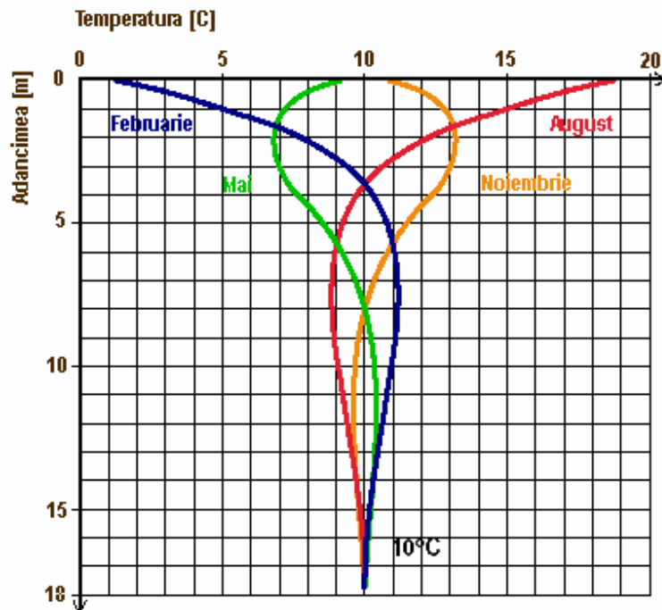
Fig. 7. Variația temperaturii în sol, în zona de la suprafața scoarței terestre www.viessmann.com
