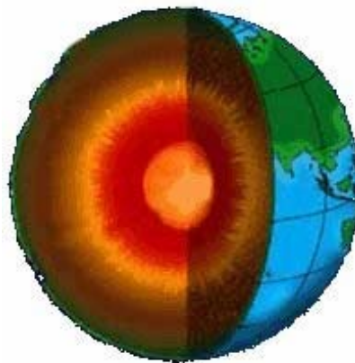
Fig. 3. Variația temperaturii în zonele din interiorul Pământului academic.evergreen.edu
